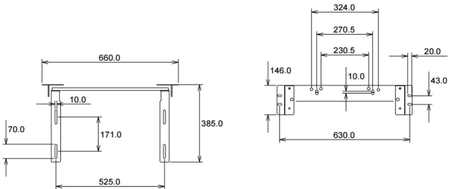
Esquema dimensional conjunto sifón
