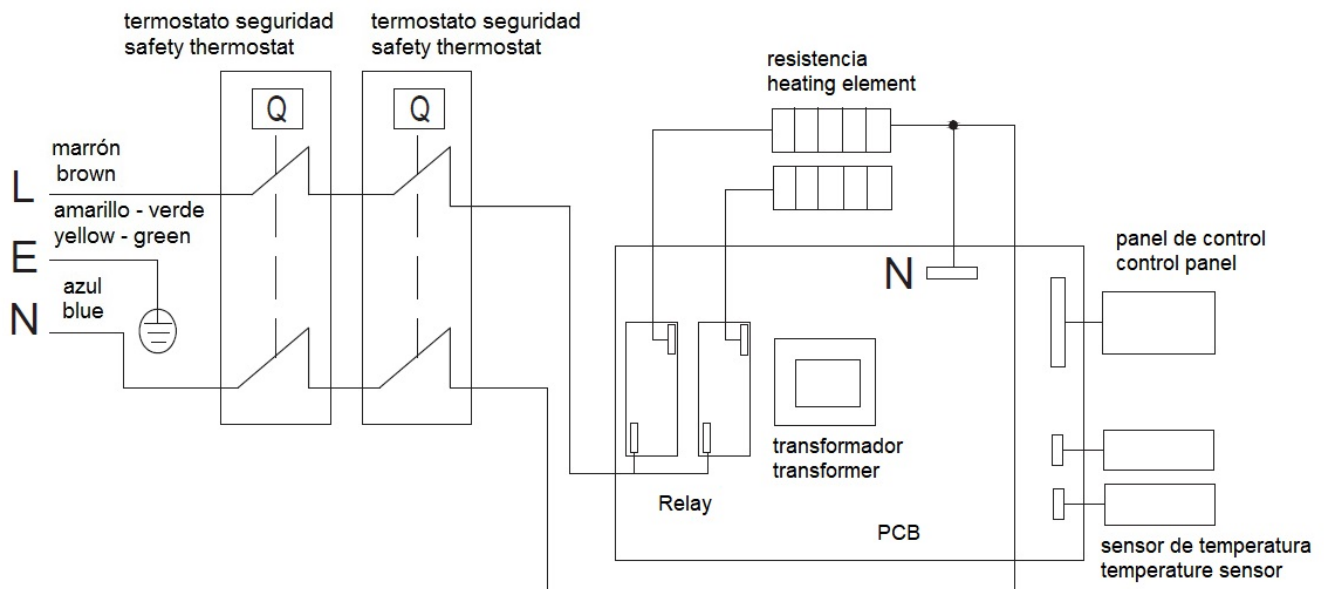
Fig. – 4 Schéma unifilaire modèle APARICI SCxxxT
