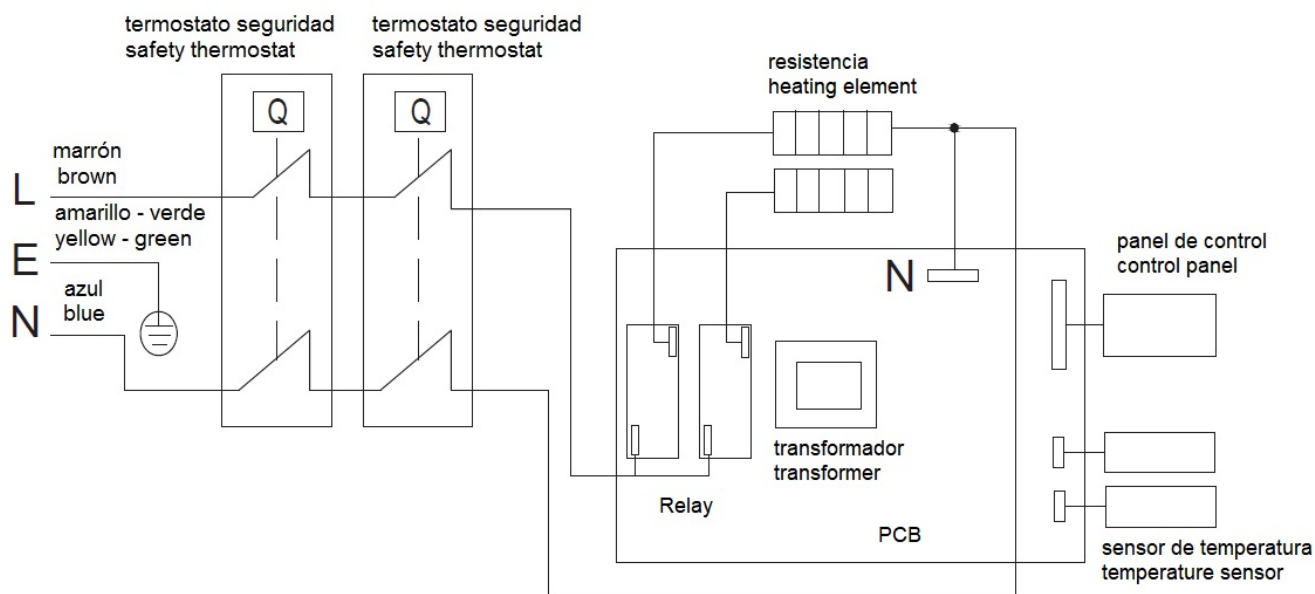
Fig. – 4 Esquema unifilar modelo APARICI – SCxxxT
