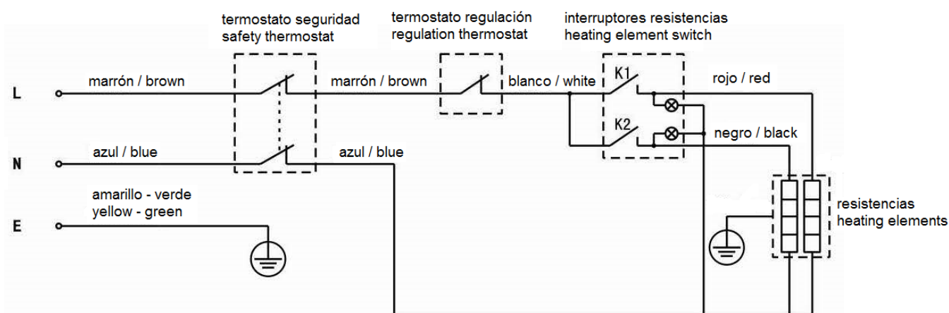
Fig. – 4 Esquema unifilar modelo NOFER – SC
